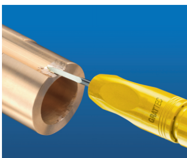
ADJUSTABLE MINI SCRAPER YT1100GT
