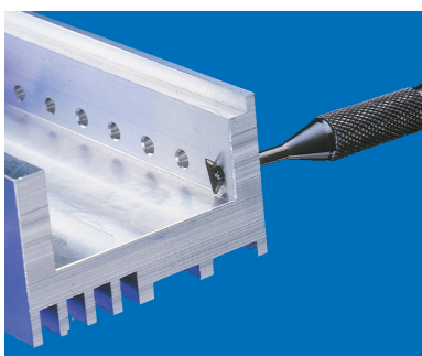
MINI REVERSIBLE COUNTERSINK RC1000GT Patented
